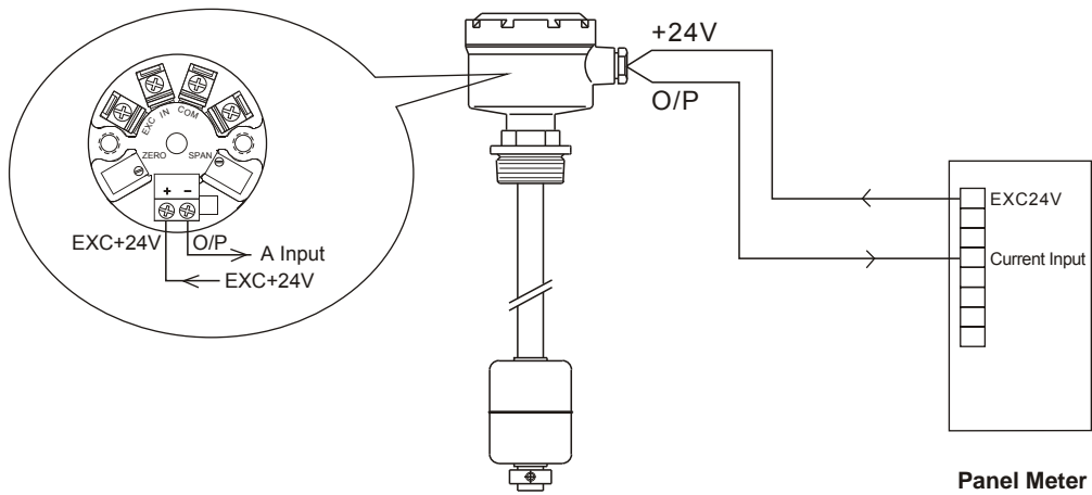
2-Wire ( RAB-2110)
